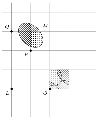
Figure 1: Décomposition M \cap S_L
